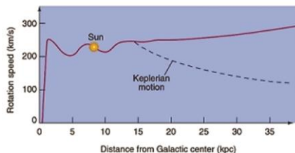
Рис.3.7 Фактическая кривая вращения и движение по Кеплеру [12]
