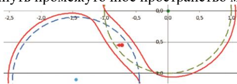
Рис.3.5. Две сверхмассивные Черные дыры разошлись и образовали тоннель убегающего
