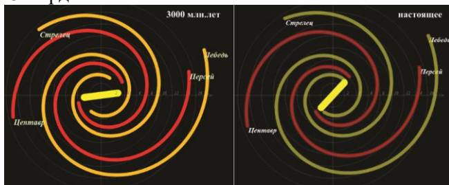
Рис.б.3 Изображение галактики Млечный Путь с рукавами, образованными за 3 млрд. лет из двух пар джетов (слева) и нынешнее её представление (справа). Кривая вращения – выпрямляющая Рукав Лебеда.
