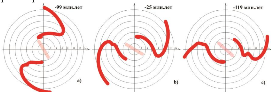
Рис.3.18 Возможно, так выглядела галактика Млечный Путь в указанное время t , когда рукава находились в промежуточном состоянии закрученности между прямым (нынешним) и обратным (предполагаемым) направлением в зависимости от кривой вращения
