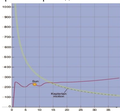
Рис.3.11 Аппроксимация кеплеровской кривой вращения рис.3.7
