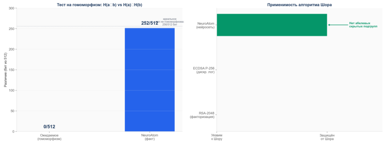
Рис. 1 Тест на гомоморфизм и применимость алгоритма Шора.
