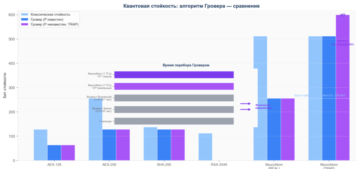
Рис. 2 Сравнение квантовой стойкости к алгоритму Гровера. Для TRAP-режима без знания открытого текста оракул не определён ( \infty ). Врезка: оценка времени перебора.
