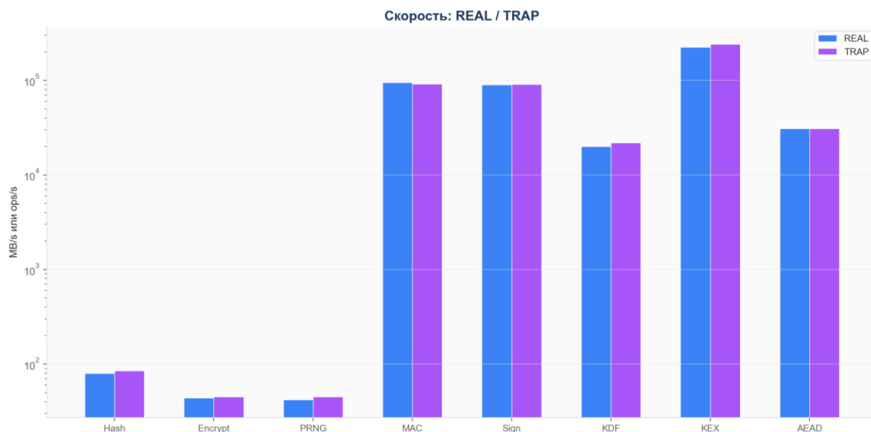
Рис. 9 Скорость операций в режимах REAL и TRAP. Логарифмическая шкала.
